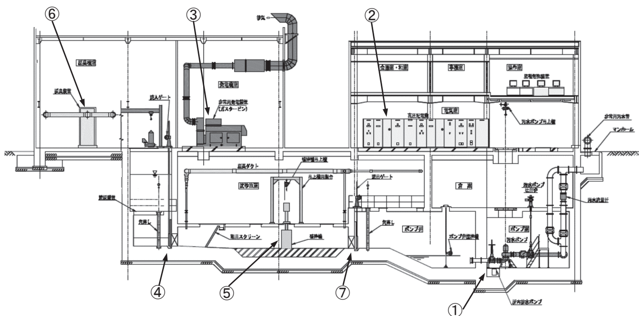
断面図
