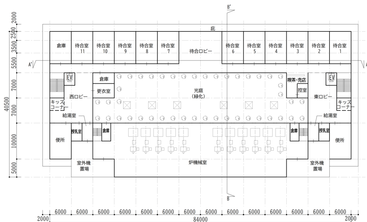
図 1-15 火葬・待合棟3階平面図（イメージ）
