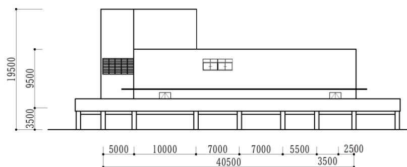
図 1-19 火葬・待合棟東側立面図（イメージ）
