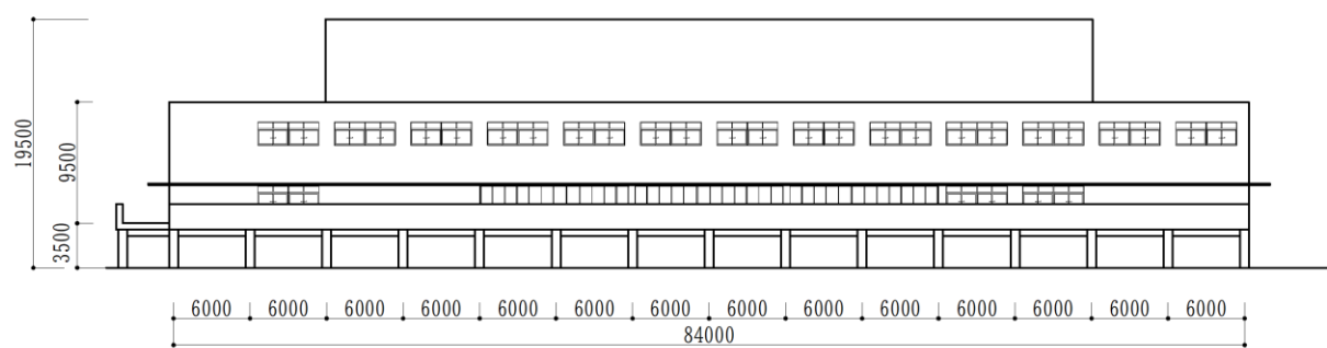
図 1-16 火葬・待合棟北側立面図（イメージ）
