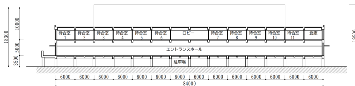
図 1-20 A-A' 火葬・待合棟断面図（イメージ）
