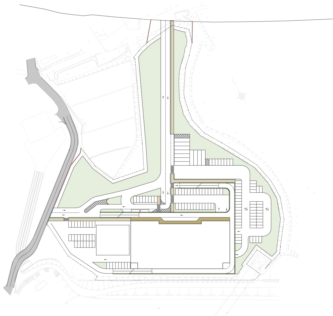
図 1-12 2階配置図（イメージ）
