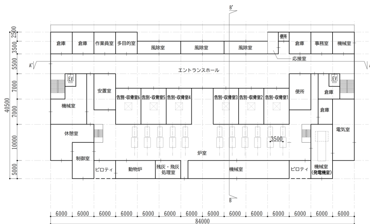
図 1-14 火葬・待合棟 2 階平面図 (イメージ)
