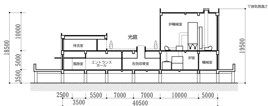
図 1-21 B-B' 火葬・待合棟断面図（イメージ）
