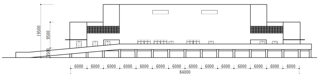
図 1-17 火葬・待合棟南側立面図（イメージ）
