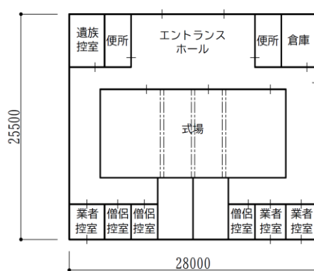
図 1-13 式場棟1階平面図（イメージ）
