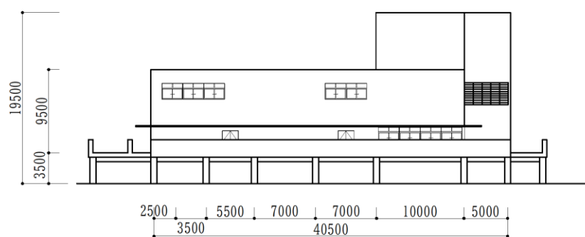
図 1-18 火葬・待合棟西側立面図（イメージ）
