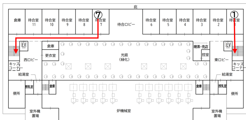
火葬・待合棟 3階平面図 (イメージ)
