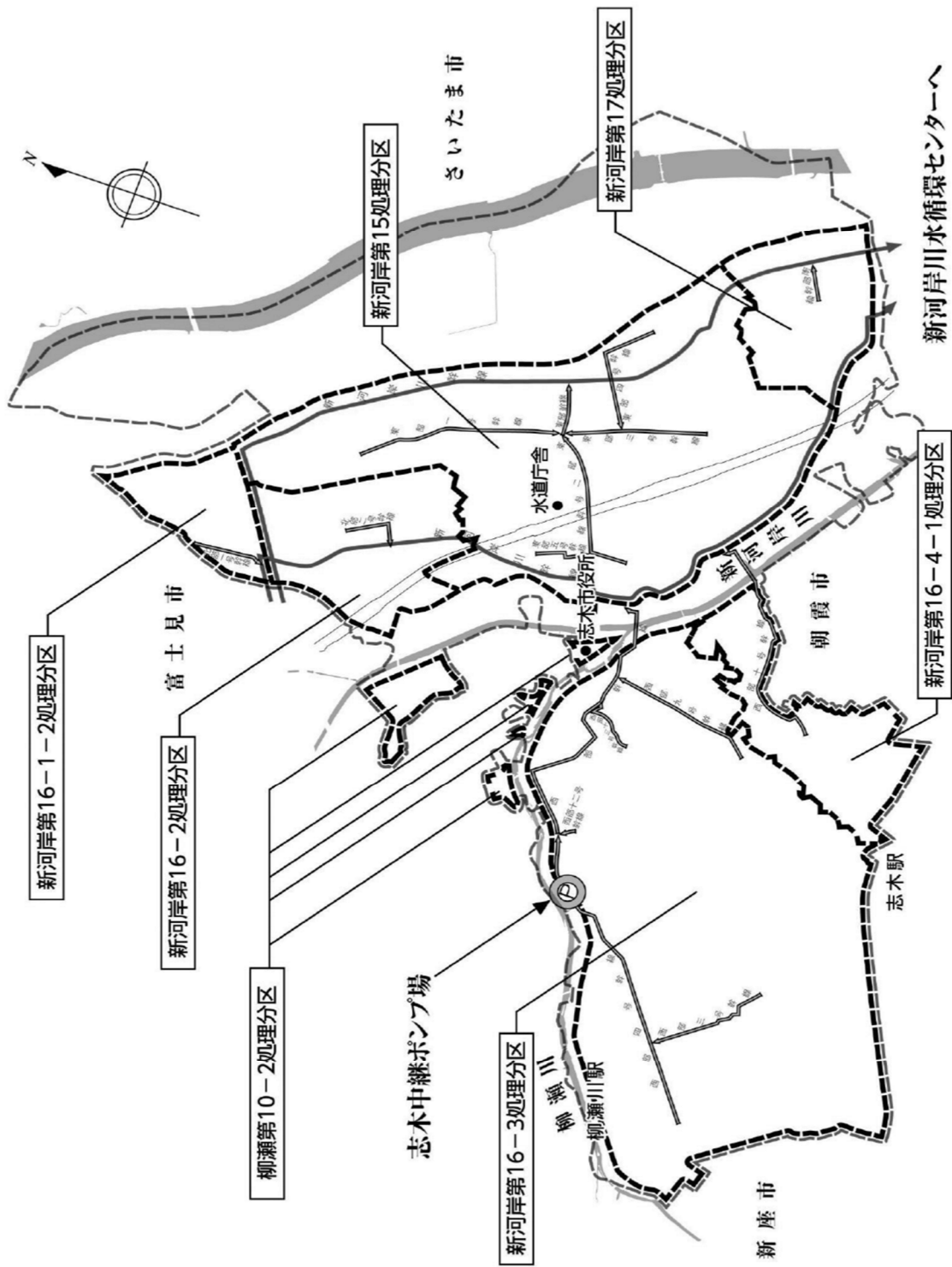
下水道処理区域（污水）
