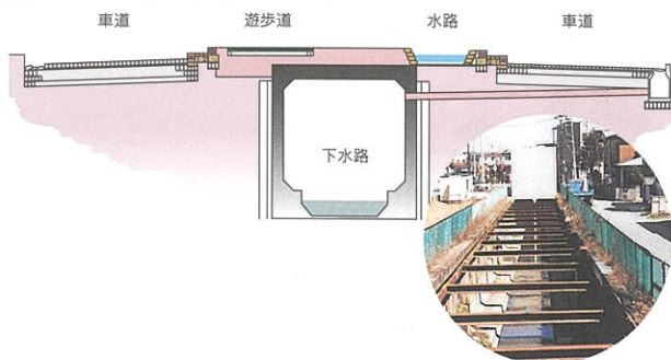
■せせらぎの小径断面図
