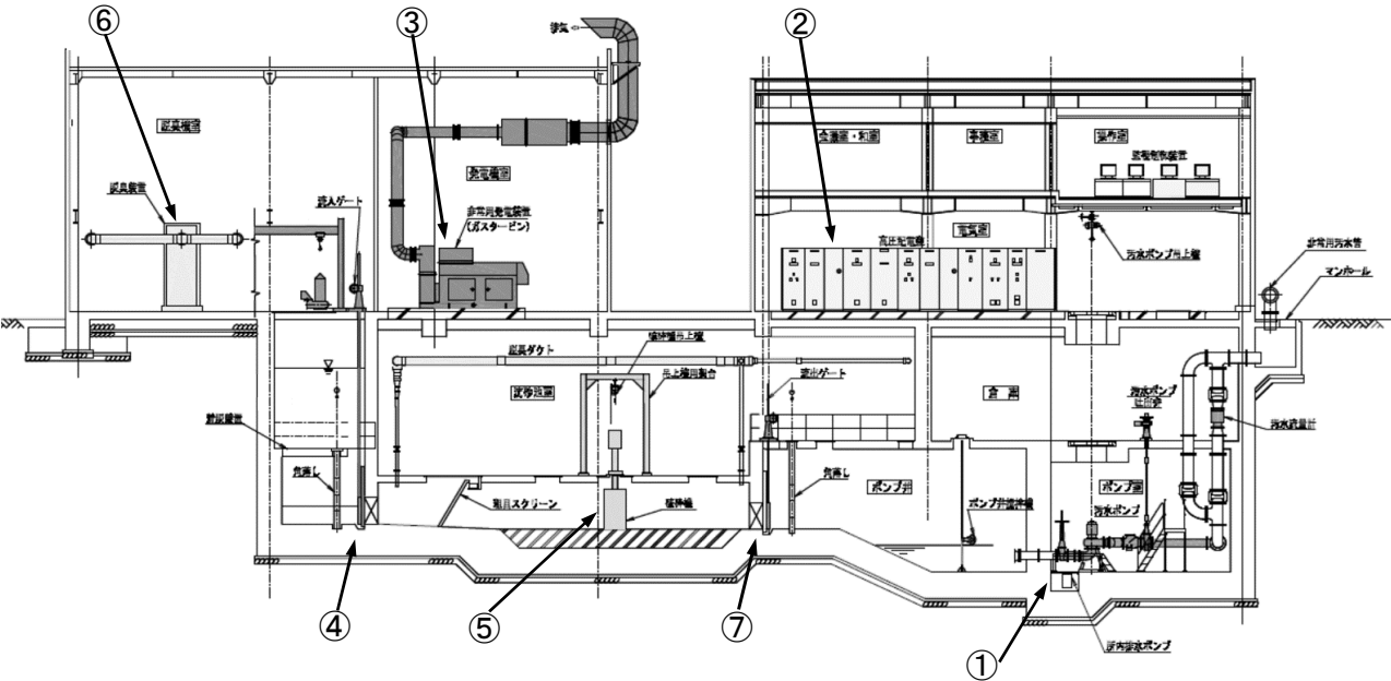
断面図
