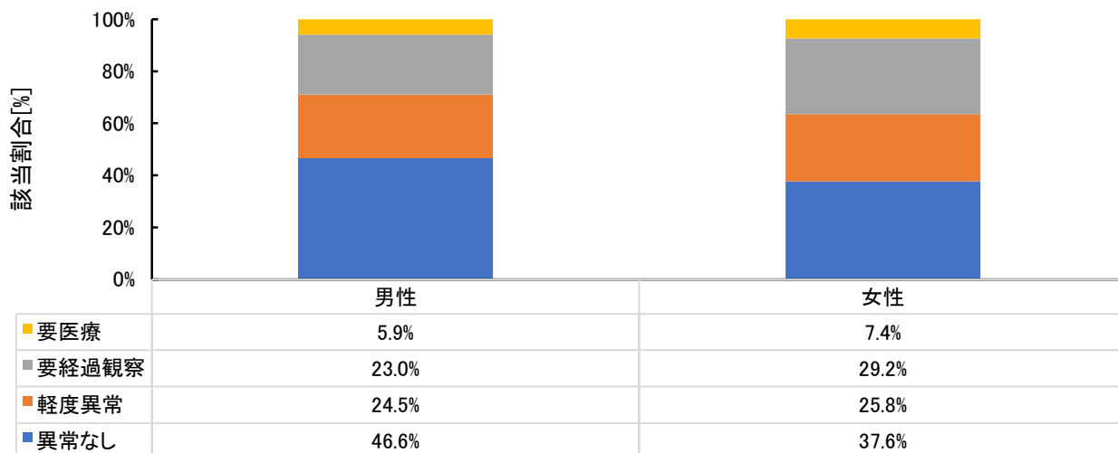
図 7-47 LDL コレステロール判定の結果
